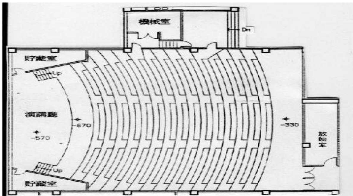
臺中市立大墩文化中心演講廳平面圖
